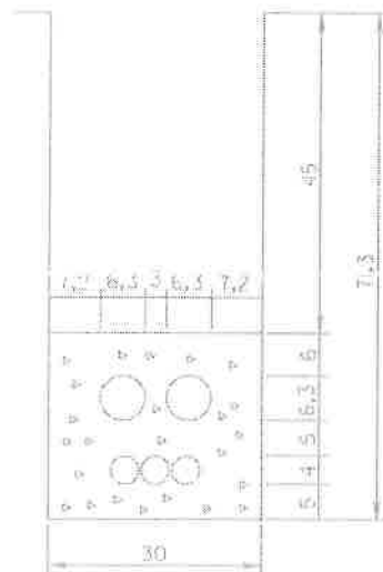
2 dia. 63 y 11ritubo NUEVOS PRISMAS DE CANALIZACION
